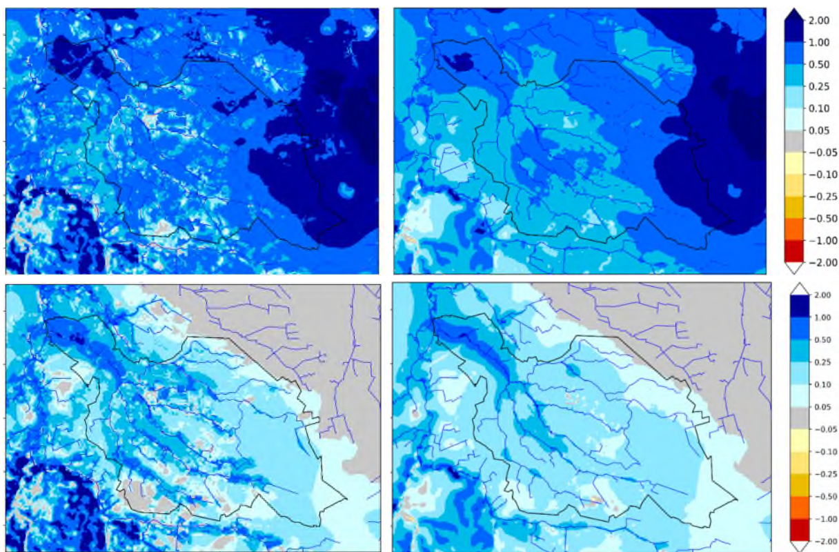
Figuur 2-7. Verandering van de GHG (links) en GLG (rechts) bij variant 'maximaal vasthouden' (1C; boven) en variant 'natuur versterken' (2B). Een blauwe kleur geeft een stijging van de grondwaterstand aan, een gele tot rode kleur geeft een daling aan. De grondwaterkarakteristieken zijn berekend over de periode 1996 – 2004. Figuren en simulaties afkomstig uit Schoonderwoerd e.a. (2022).
