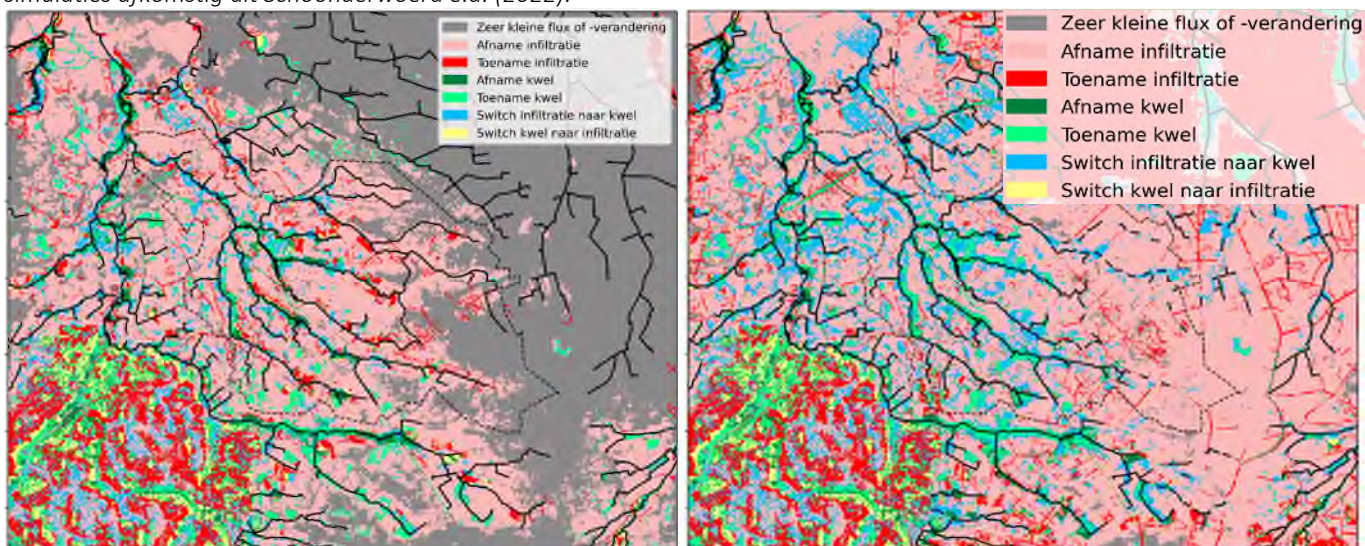
Figuur 2-8. Verandering jaargemiddelde kwel bij V2B Maximaal vasthouden (links) en V1C (rechts) ten opzichte van de referentie bij WH 2050. Kaarten afkomstig uit Schoonderwoerd e.a. (2022).
