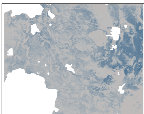
Figuur 3-13. Met PROBE gesimuleerde transpiratiestress (bovenste rij) en verandering ervan ten opzichte van het scenario met enkel klimaatverandering (onderste rij) bij de twee inrichtingsvarianten. Transpiratiestress is uitgedrukt als de maximale jaarlijkse transpiratiereductie (verschil actuele en potentiële transpiratie voor een referentiegras) gedurende 10 dagen, gemiddeld over een periode van 30 jaar (mm water).
