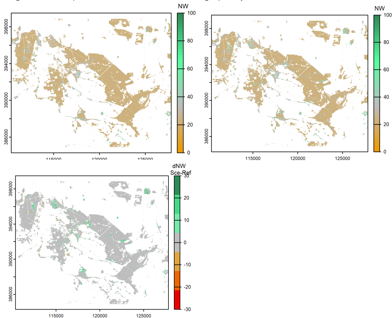
Figuur 3-10. Natuurwaarde (0 – 100) bij huidig klimaat (linksboven) en toekomstig klimaat (rechtsboven) voor huidige natuur; zichtjaar 2050, scenario 0B, en het berekende verschil (scenario – referentie) voor houtige vegetaties (onder).
