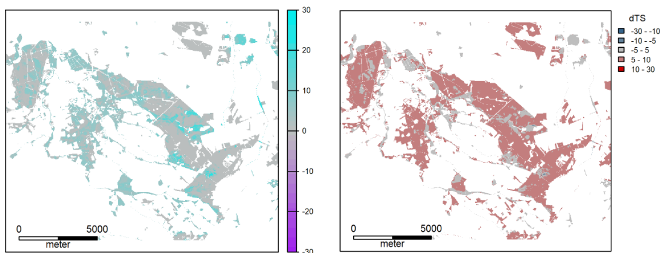
Figuur 3-5. Door PROBE voorspelde verandering in zuurstofstress (links) en transpiratiestress (rechts) als gevolg van klimaatverandering. Zie bijschrift Figuur 3-4 voor toelichting.
